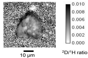
図1 重水素/水素比(2D/1H)をマーカーにしたジェオスミンの活性炭内吸着量分布
